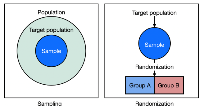
ภาพที่ 1 แผนภาพเปรียบเทียบการสุ่มตัวอย่าง (Sampling) และการสุ่มแบ่งกลุ่ม (Randomization)
