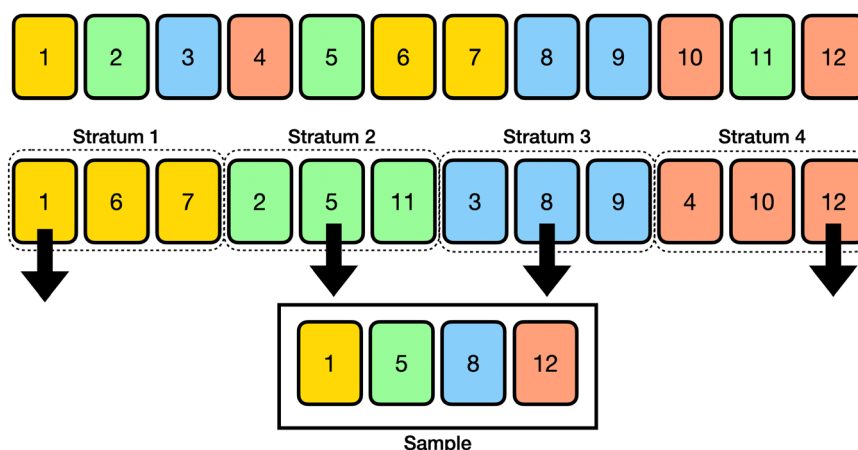
ภาพที่ 3 แผนภาพการสุ่มตัวอย่างแบบแบ่งชั้น (Stratified Sampling)
