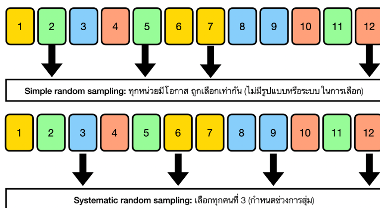
ภาพที่ 2 แผนภาพการสุ่มตัวอย่างแบบง่าย (Simple Random Sampling) และการสุ่มตัวอย่างแบบมีระบบ (Systematic Sampling)
