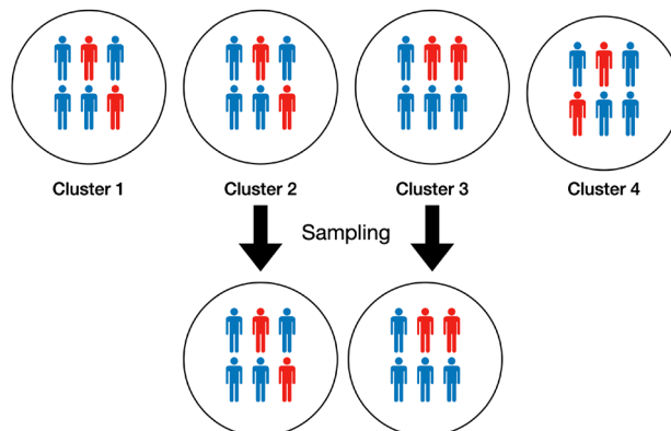
ภาพที่ 4 แผนภาพการสุ่มตัวอย่างแบบกลุ่ม (Cluster Sampling)
